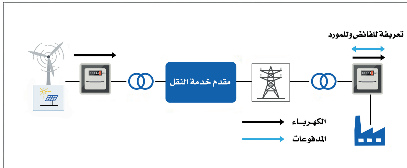
الشكل (٧): استهلاك ذاتي افتراضي عبر شبكة النقل، توليد واحد، وموقع استهلاك واحد
