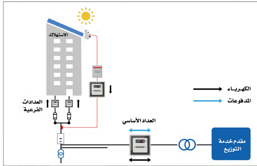
الشكل (٦): استهلاك ذاتي مشترك في الموقع
