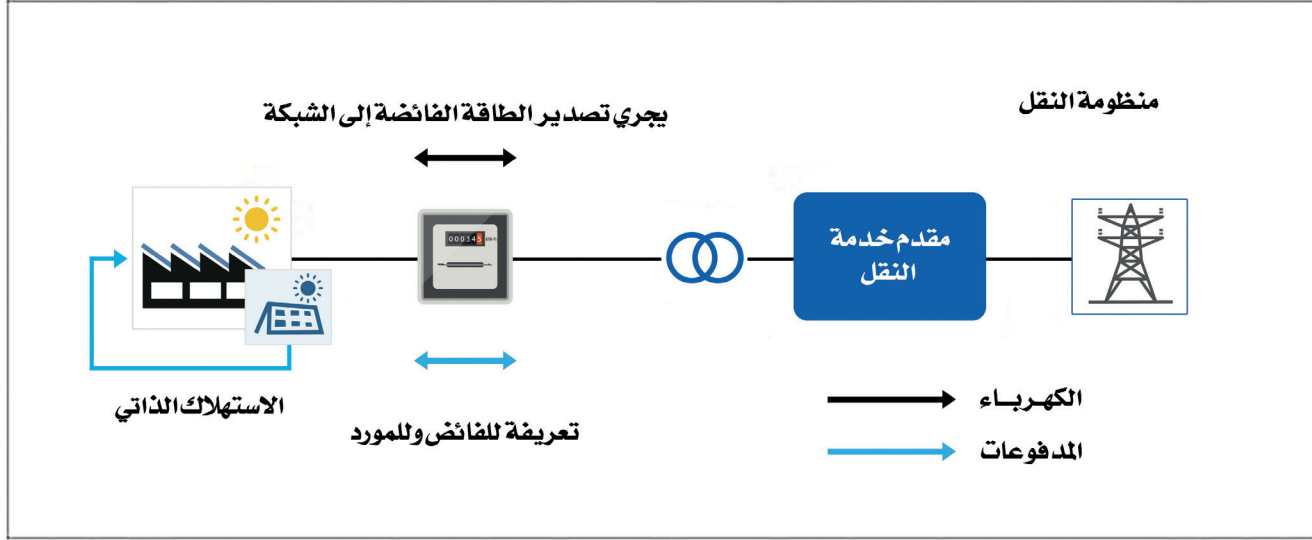
الشكل (٥): استهلاك ذاتي في المنشأة بطاقة فائضة مرتبط بشبكة النقل
