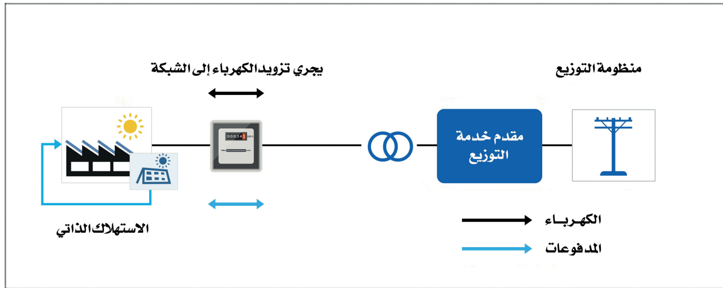
الشكل (3): استهلاك ذاتي في المنشأة بطاقة فائضة مرتبط بشبكة التوزيع
