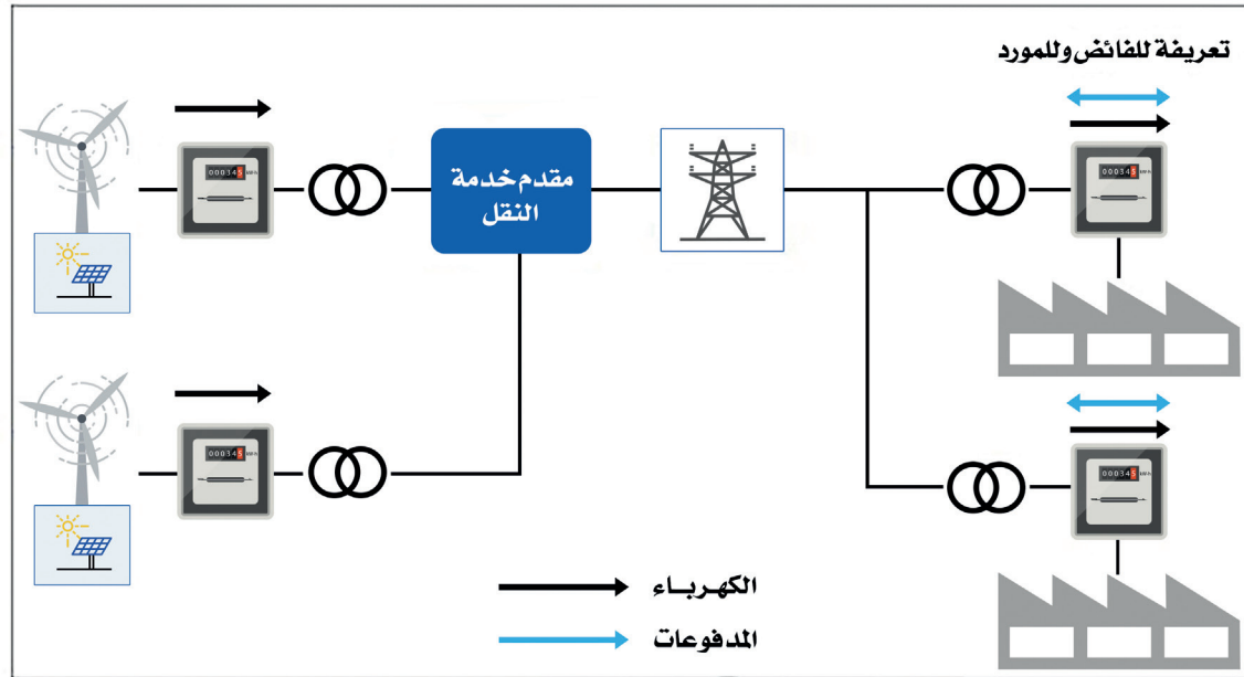
الشكل (٨): استهلاك ذاتي افتراضي عبر شبكة النقل، منظومات توليد عديدة و/أو مواقع استهلاك عديدة
