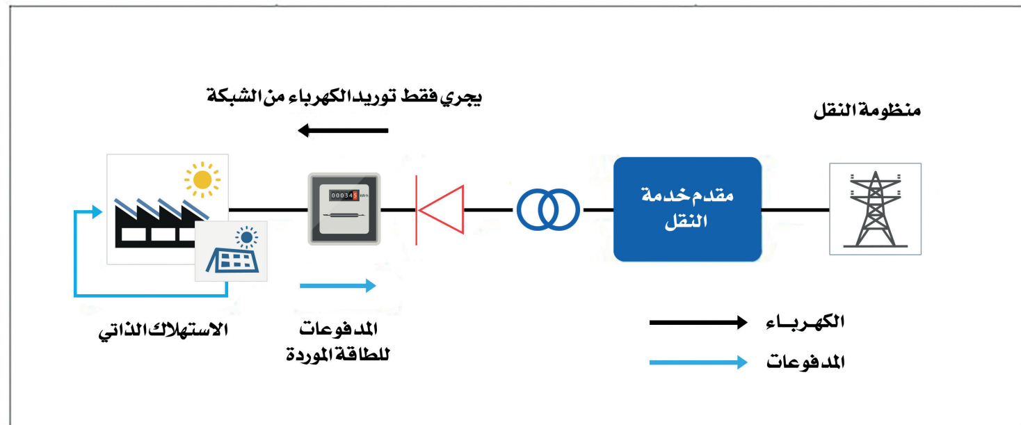
الشكل (4): استهلاك ذاتي في المنشأة دون ترحيل مرتبط بشبكة النقل
