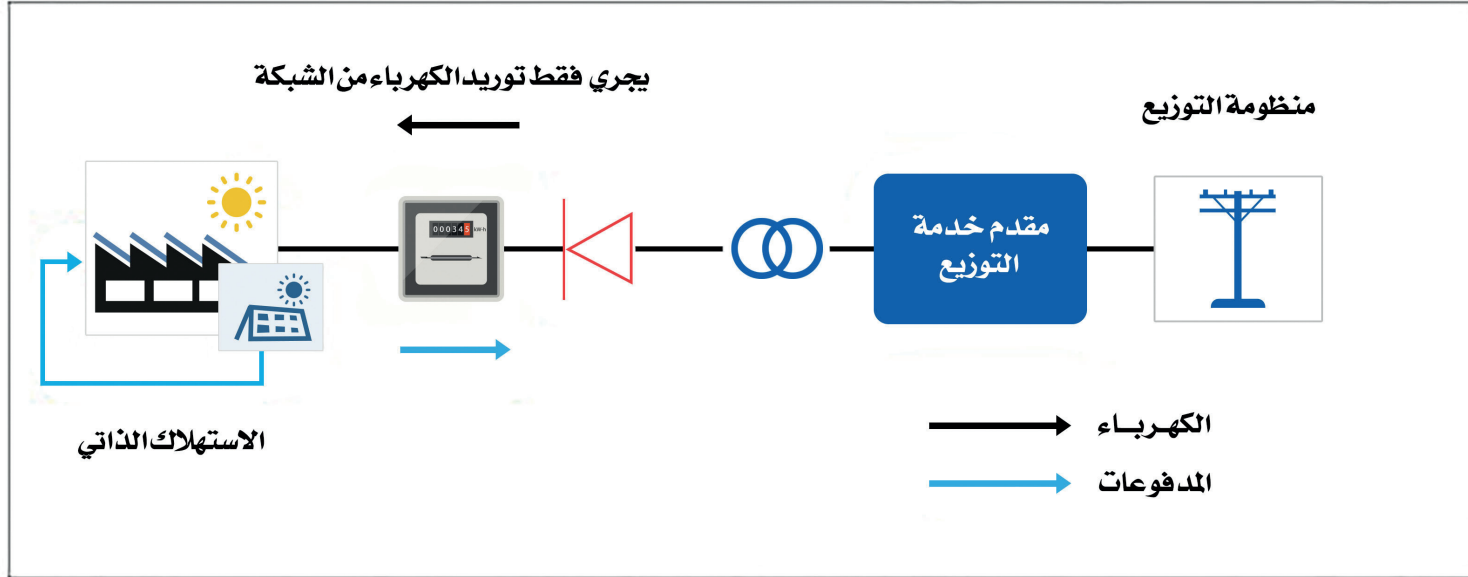
الشكل (2): استهلاك ذاتي في المنشأة دون ترحيل مرتبط بشبكة التوزيع
