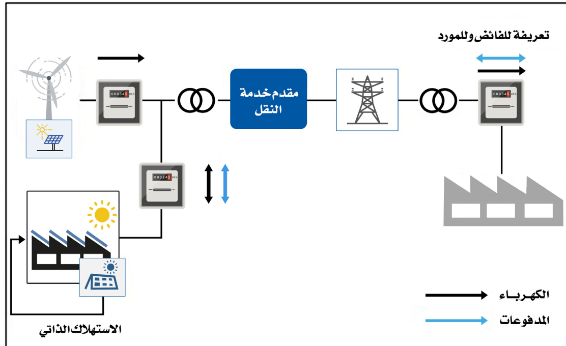
الشكل (٩): استهلاك ذاتي في الموقع وافتراضي عبر شبكة النقل، منظومات توليد عديدة، ومواقع استهلاك عديدة
